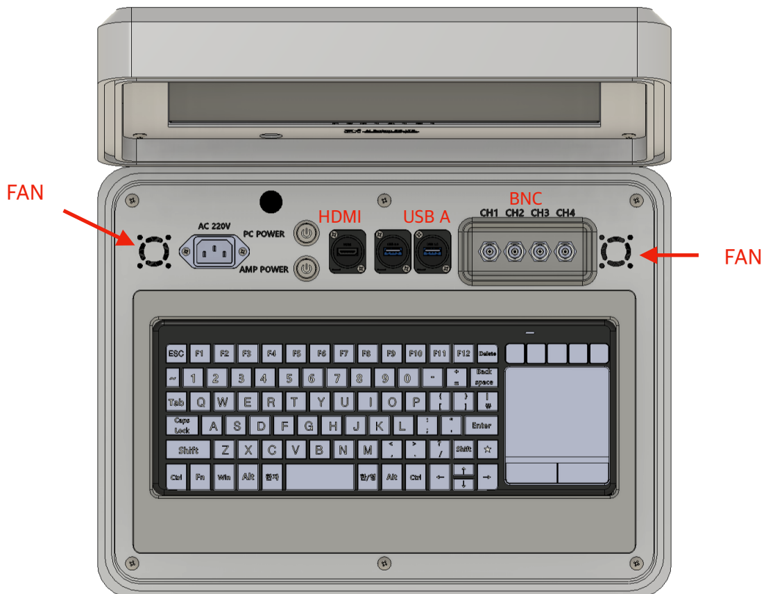
[ 포터블 측정기 주요 부위 명칭 ]
